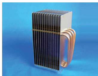
■ヒートパイプ式ヒートシンク
