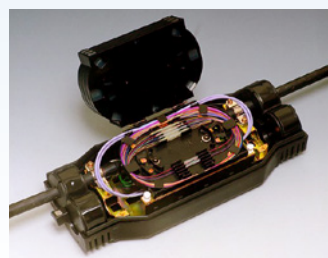
■光ケーブルクロージャ
