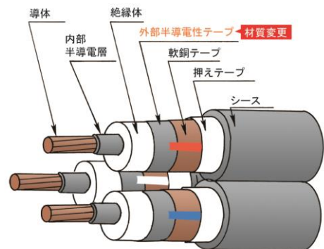
図1 高圧(6600V)ケーブルの構造
